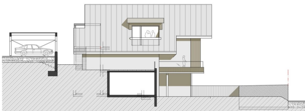
Schnittansicht B-B Süd-West M:1:100
