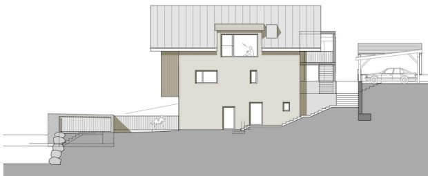
Ansicht Nord-Ost M:1:100
